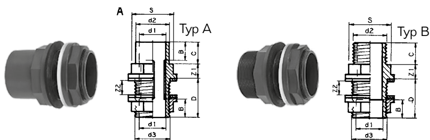
Durchführung mit Klemmutter Transition avec écrou autobloquant
