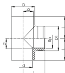
Art. Nr. 27.20.02 T-Stück 90°, Abgang mit IG
